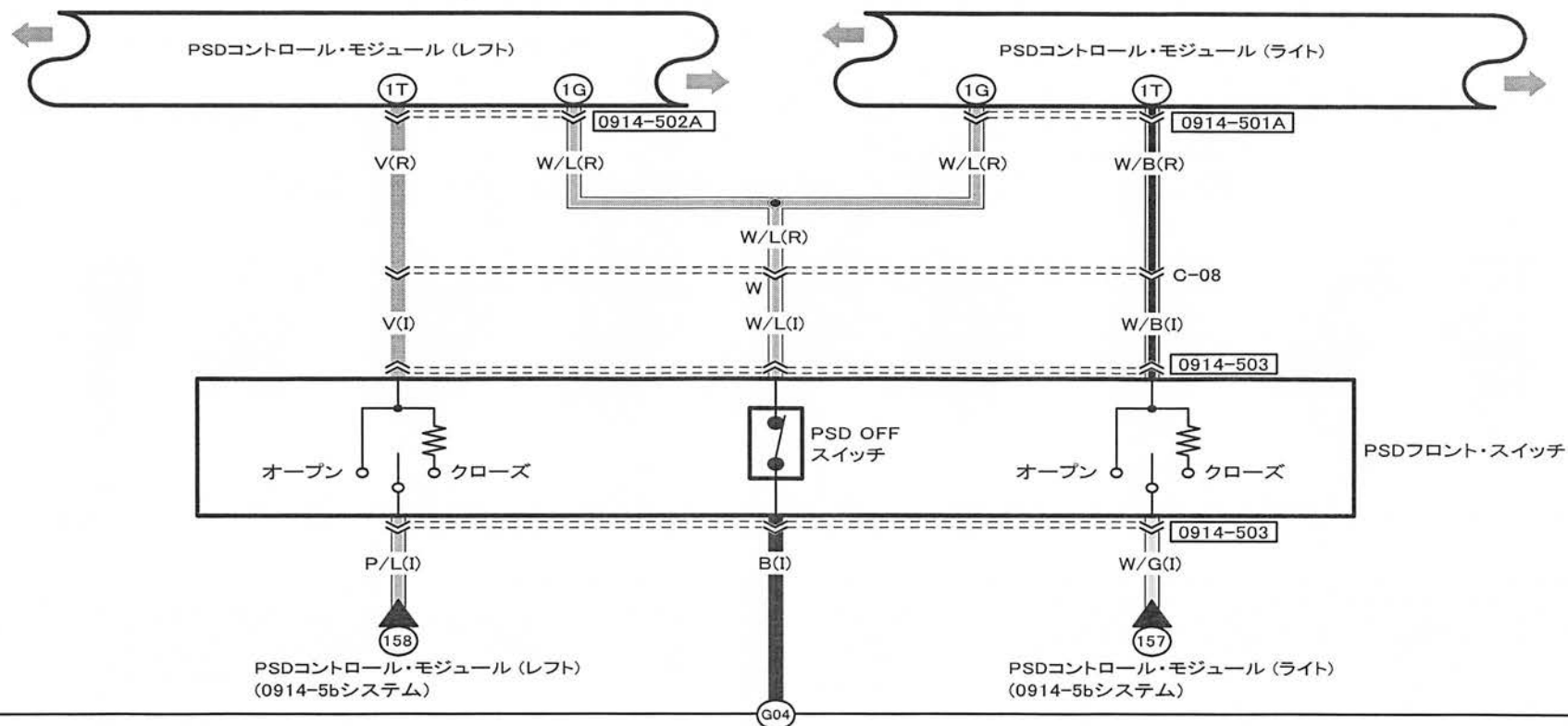
0914-501A PSDコントロール・モジュール (右)
