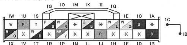
0914-502A PSDコントロール・モジュール (レフト)
