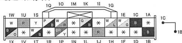
0914-502A PSDコントロール・モジュール (レフト)
