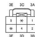
0914-502C PSDコントロール・モジュール (レフト)
