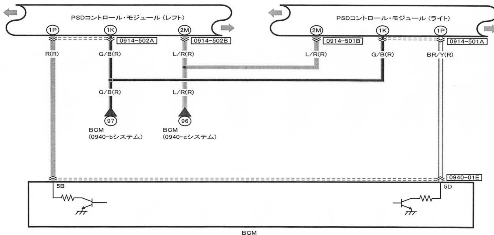
0914-501A PSDコントロール・モジュール (ライト)
