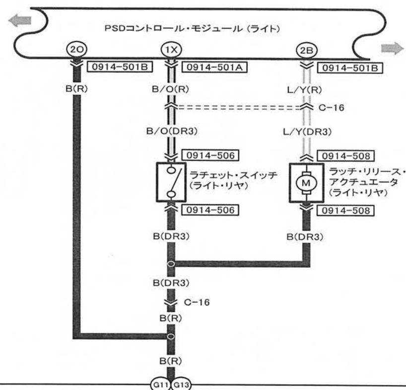
0914-501B PSDコントロール・モジュール (ライト)
