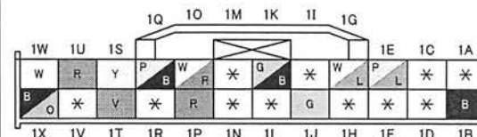
0914-502A PSDコントロール・モジュール (レフト)
