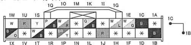
0914-501B PSDコントロール・モジュール (ライト)
