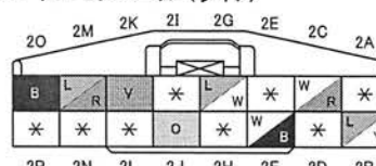
0914-502B PSDコントロール・モジュール (レフト)
