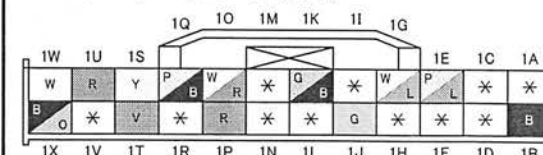
0914-508 ラッチ・リリース・ アクチュエータ (ライト・リヤ)
