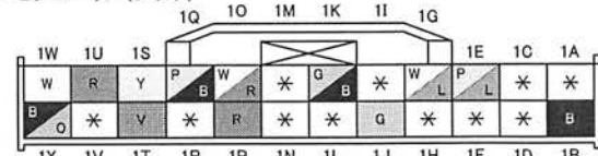
0914-502A PSDコントロール・モジュール (レフト)
