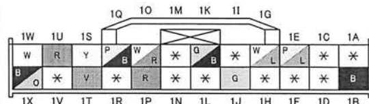
0914-502A PSDコントロール・モジュール (左)
