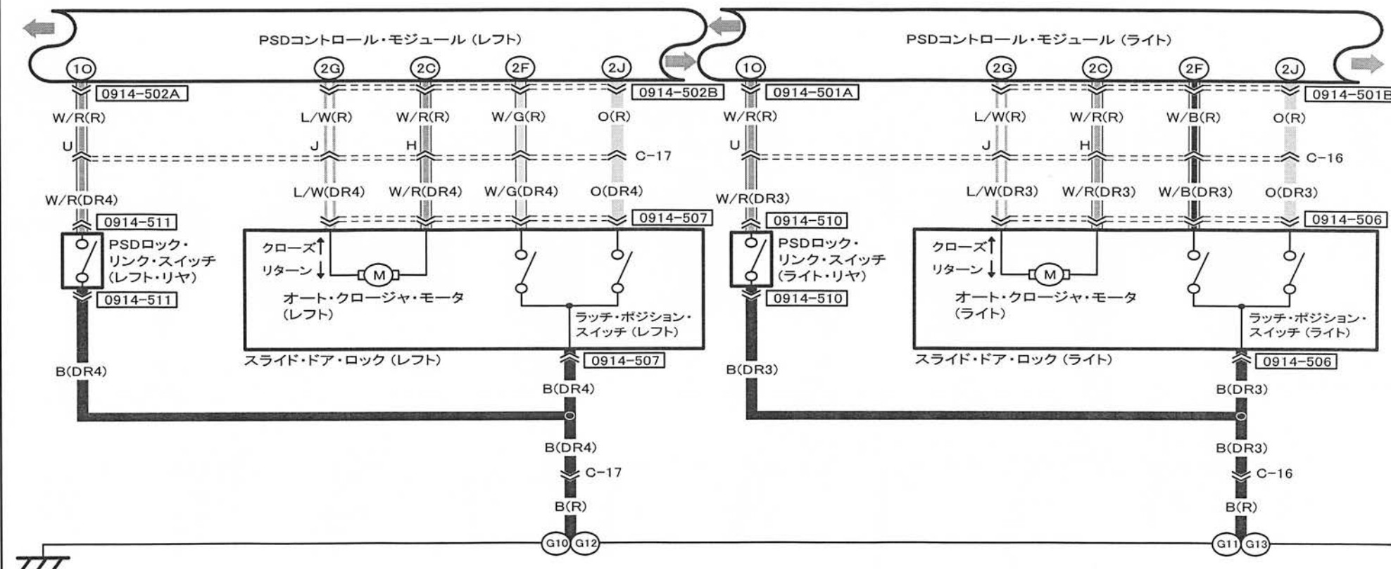
0914-501B PSDコントロール・モジュール (ライト)
