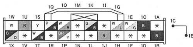
0914-502B PSDコントロール・モジュール (レフト)
