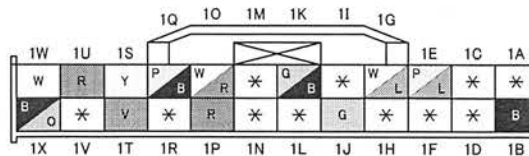
0914-502A PSDコントロール・モジュール (レフト)
