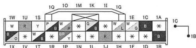
0914-501A PSDコントロール・モジュール (ライト)
