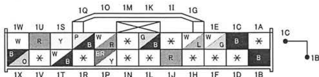
0914-501A PSDコントロール・モジュール (右)
