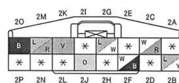
0914-506 ラチェット・スイッチ (ライト・リヤ) / スライド・ドア・ロック (ライト)
