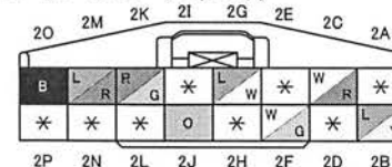
0914-502B PSDコントロール・モジュール (レフト)
